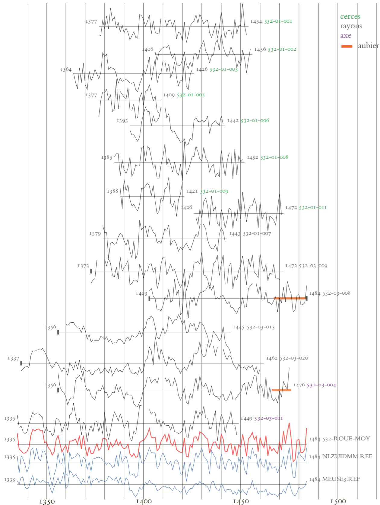
▲ Fig. 22 : séquences dendrochronologiques des bois datés, avec, en bas, la chronologie moyenne du site et deux chronologies de référence (Sud des Pays-Bas par Esther Jansma, Amersfoort et région mosane, par Patrick Hoffsummer, ULg-CEA). (ULg-CEA, 2014.)
