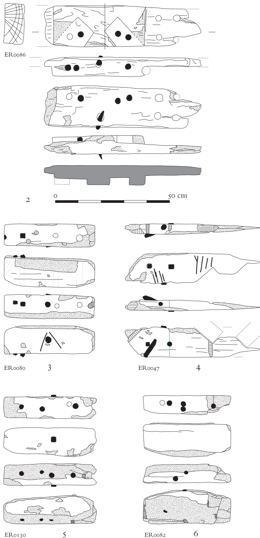
► Fig. 20-2 à 20-6 : pièces en chêne de la roue d'écureuil ; fragments d'un flasque du tambour qui recevait peut-être les rayons secondaires ; des contre-marques apparaissent sur deux des éléments. (Relevé et infographie, E. D., ULg-CEA, 2014.)
